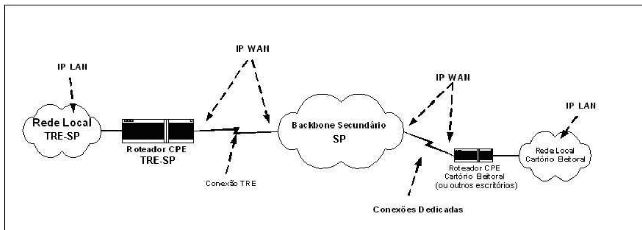
Figura 3: Localização dos IP LAN e IP WAN para conexões dedicadas
